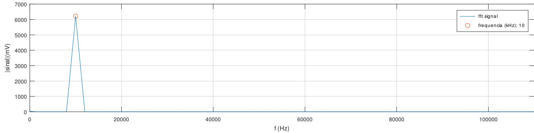
Espectro de amplitudes unilateral X(t) - Saída f=10kHz do gerador de sinais com ganho máximo
